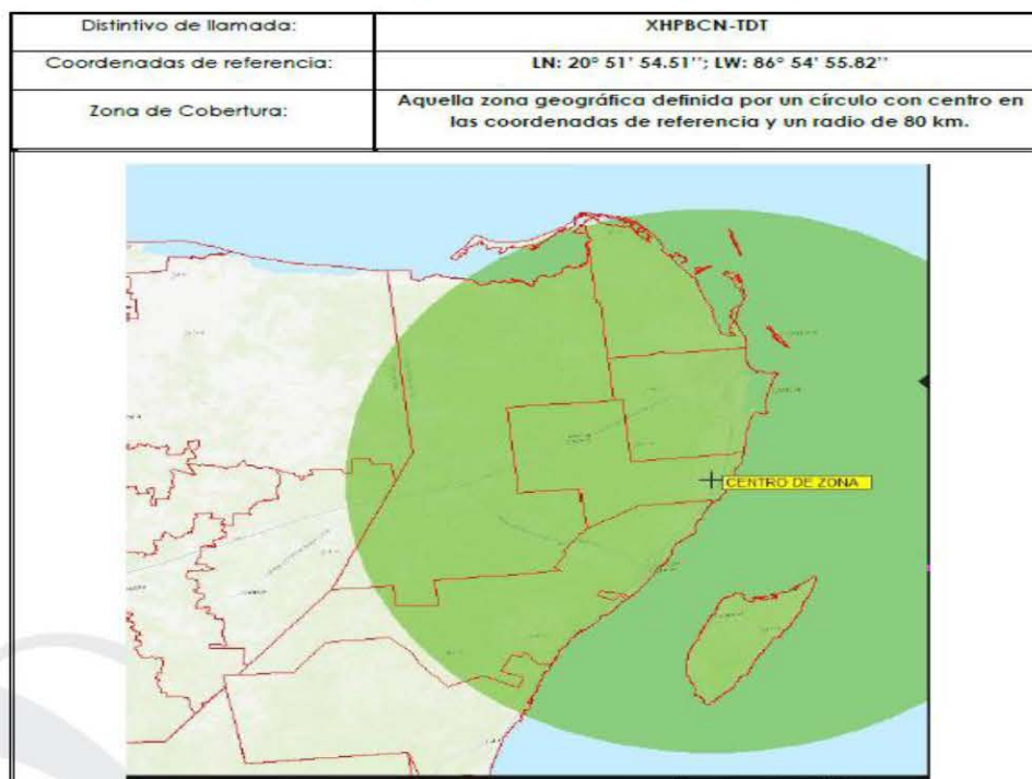
ANEXO Zona de cobertura XHPBCN-TDT en Cancún, Q. Roo
